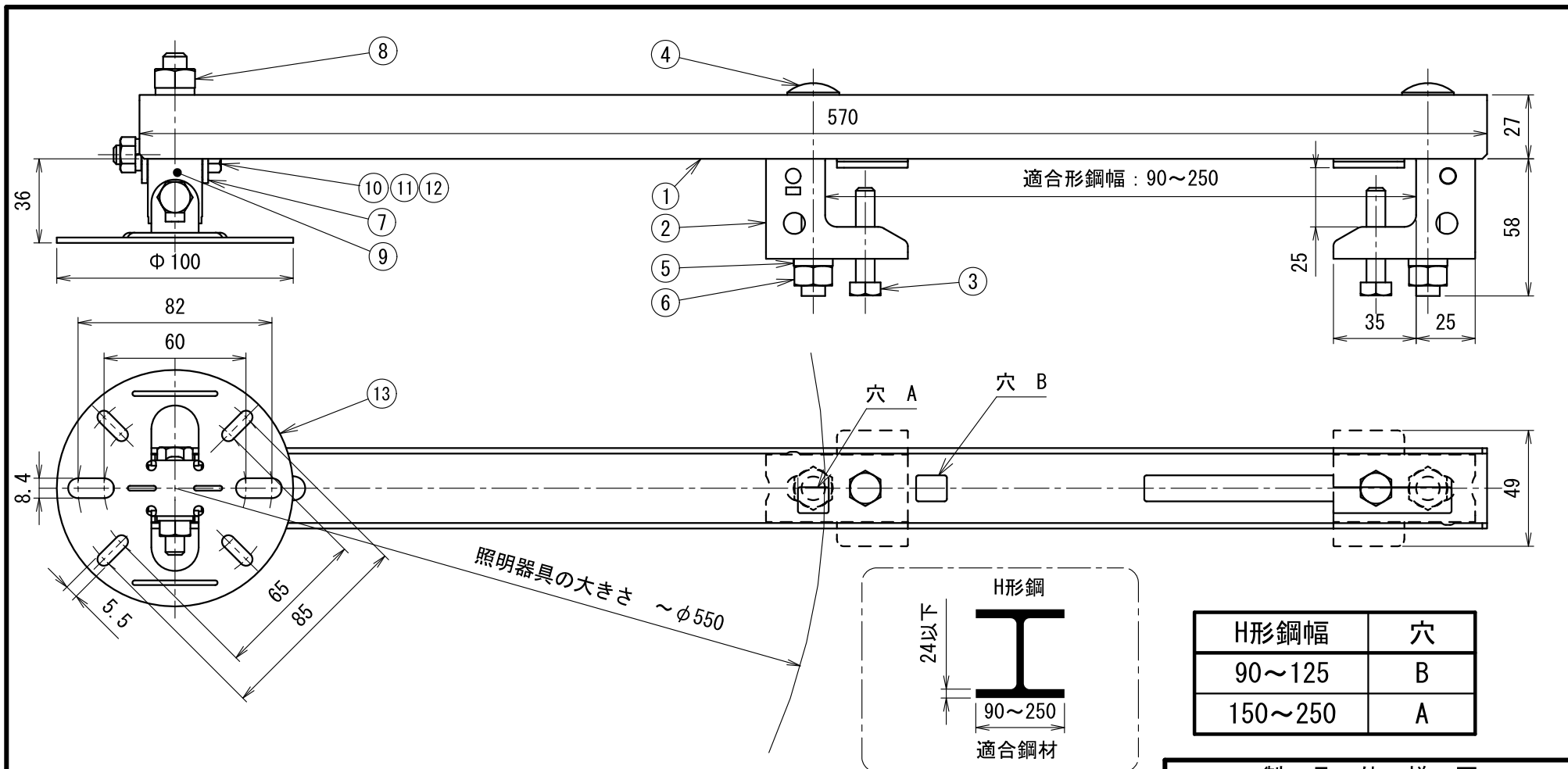
製品仕様図
